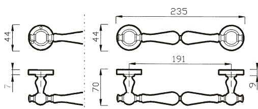
53 MNVV MANIGLIONE PULL HANDLE
