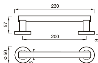
85 MN MANIGLIONE PULL HANDLE
