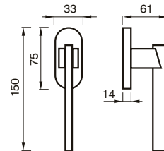
145 DK CREMONESE DK WINDOW HANDLE DK
