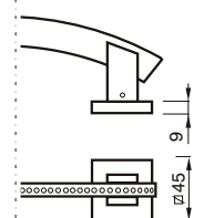
08 MNOSW MANIGLIONE PULL HANDLE
