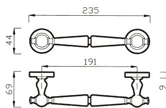
91 MN MANIGLIONE PULL HANDLE
