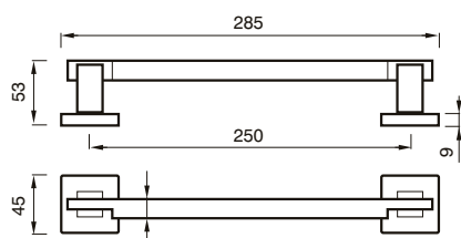
54 MN MANIGLIONE PULL HANDLE
