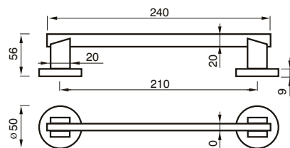
145 MN MANIGLIONE PULL HANDLE
